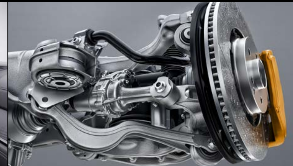
201 – Asse posteriore sterzante
