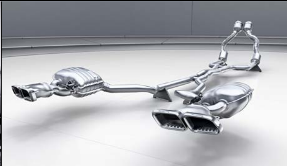
U78 – Sistema di scarico commutabile AMG Performance
