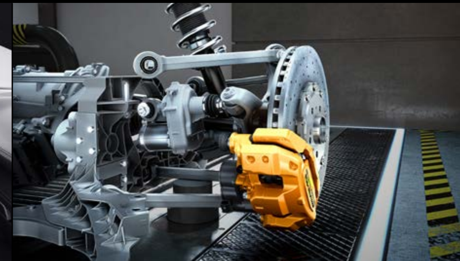
201 – Hinterachslenkung
